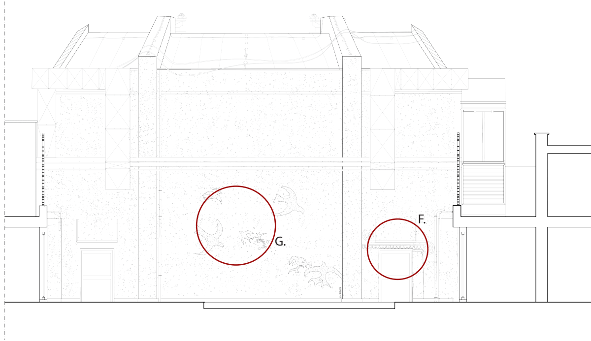
ELEVATION A-A'
